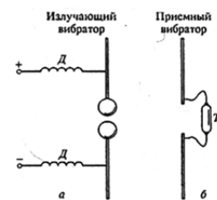
Рис. 178. Вибратор Герца
